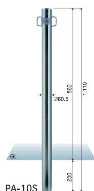
■両フック
