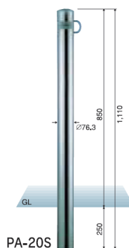
■片フック
