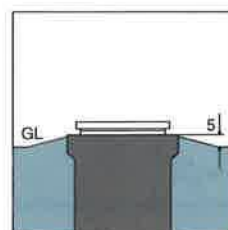
■施工時はケーシングをGLより5mm位上げて施工してください。
